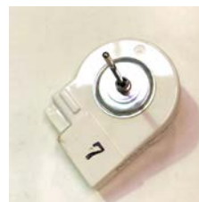
RFS911 SAMSUNG 12V FAN MOTOR (3PINS)(DA31- 00020M)
